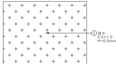
하부슬래브
